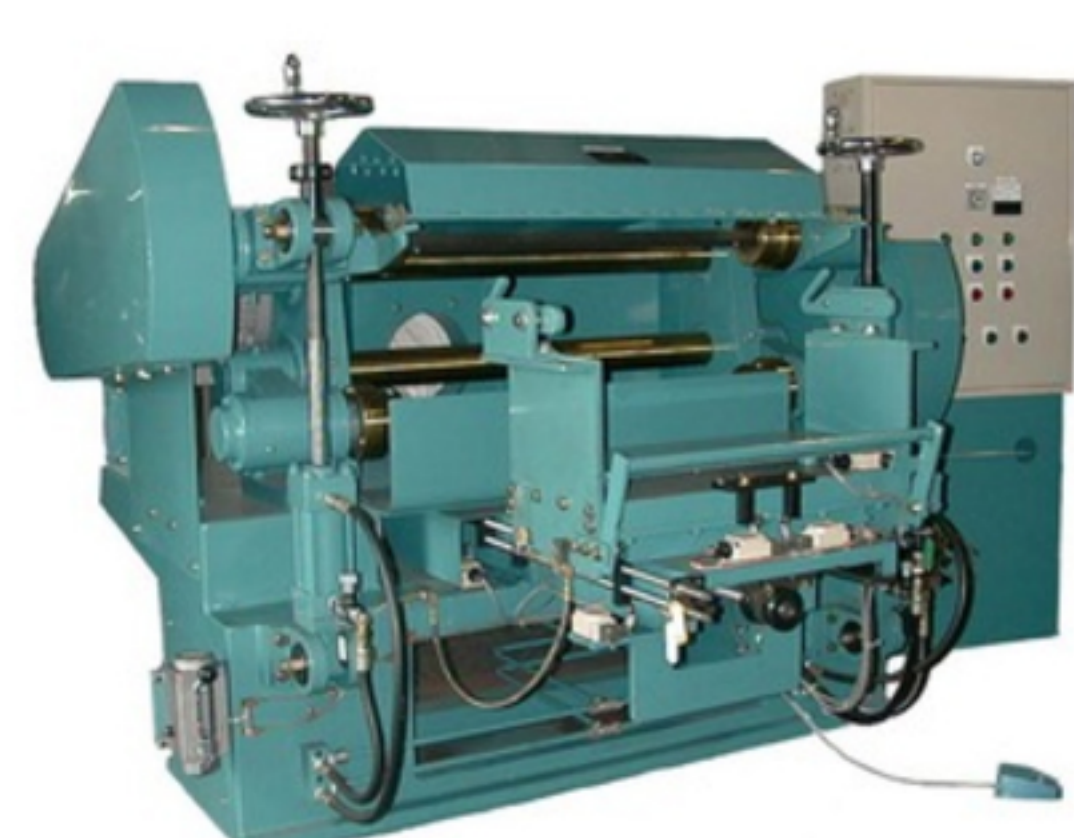
▶ 自動バフ盤
